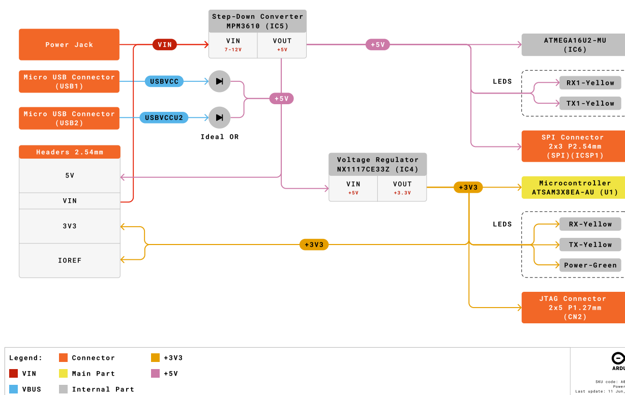
Arduino Due Power Tree
