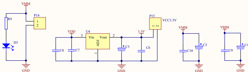
POWER_PART
