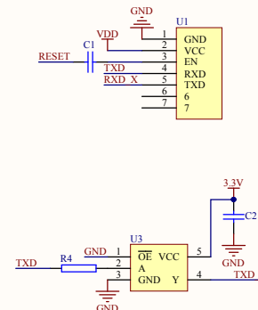
XBEE_PART
